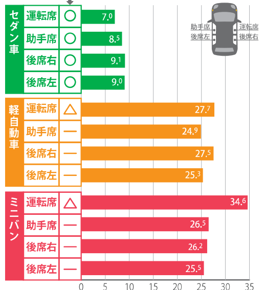
図：パワーウィンドウのスイッチを引っ張ったときの窓が閉まる力(車種と挟み込み防止機能あり・なし別)
